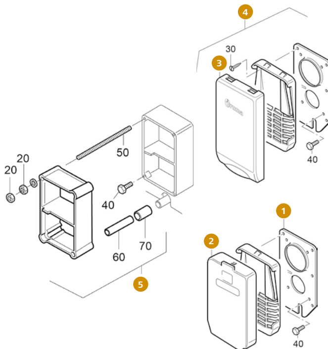
Abgasführung
